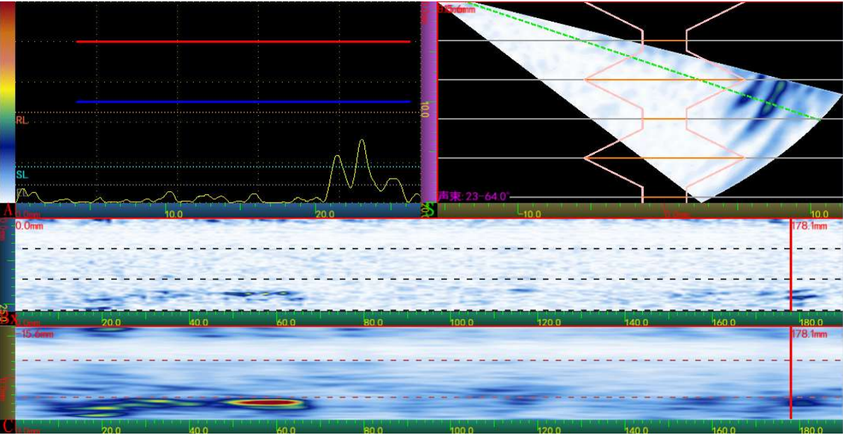
SPOOL-006 JUNTA-014
