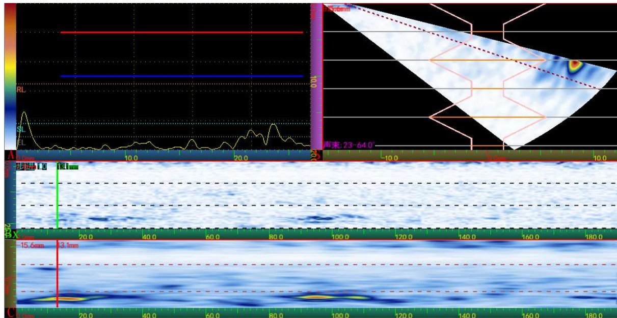
SPOOL-005 JUNTA-012
