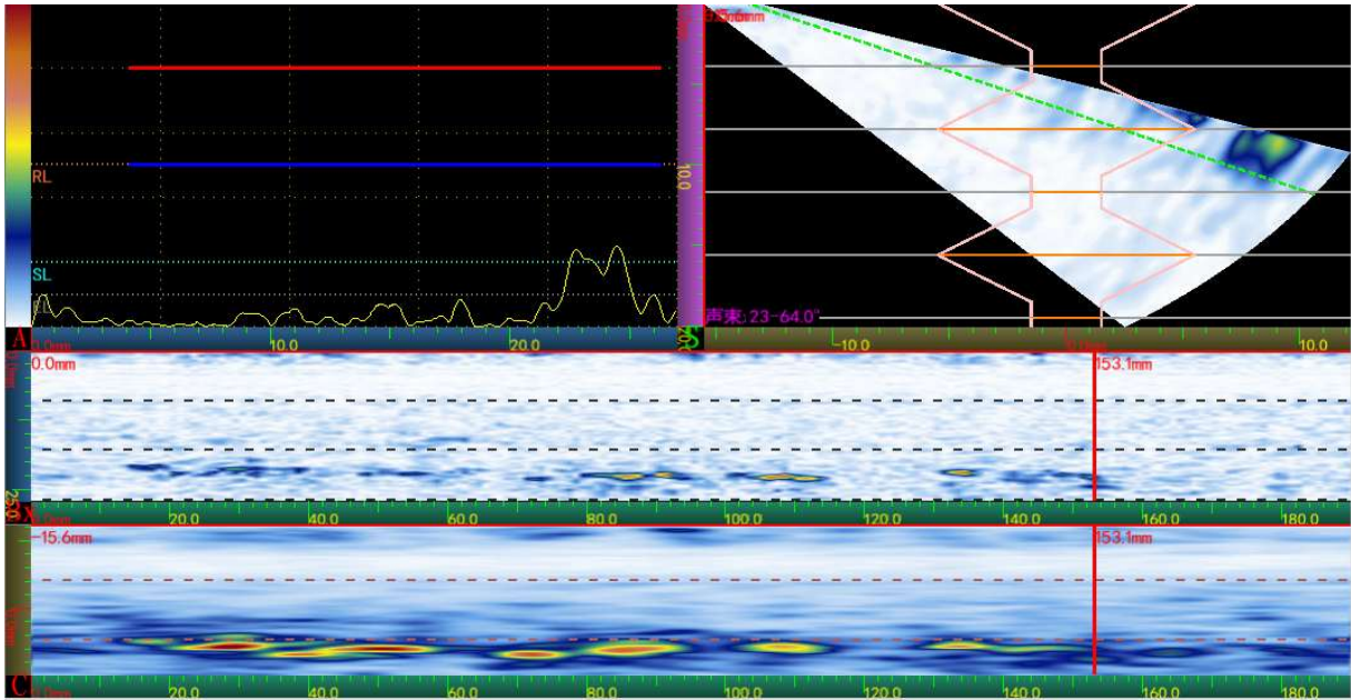
SPOOL-003 JUNTA-007
